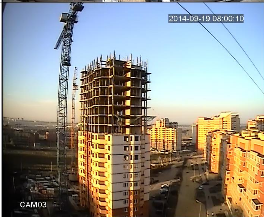
Корпус 40А. Монтаж последнего яруса колон (завершение). Монтаж 19 этажа и тех.этажа. Электротехнические работы. Штукатурные работы. Монтаж ИТП в техподполье. Прокладка теплосети от точки врезки городских коммуникаций к дому.
